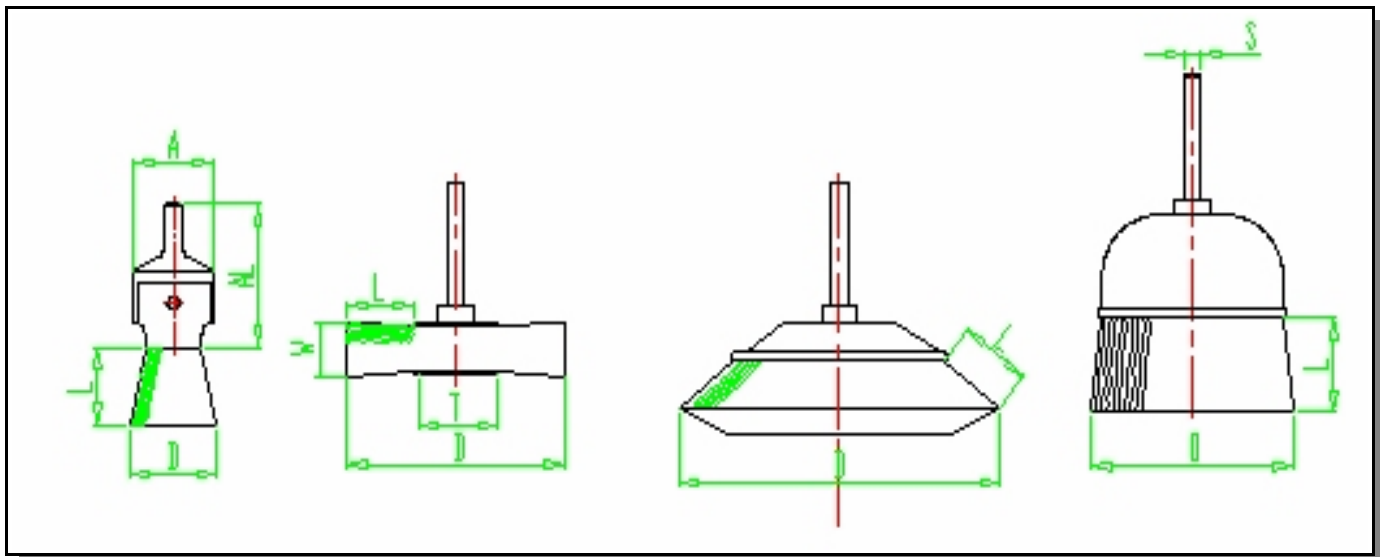
附柄鋼刷系列(所有尺寸皆可依客戶需求訂製)
