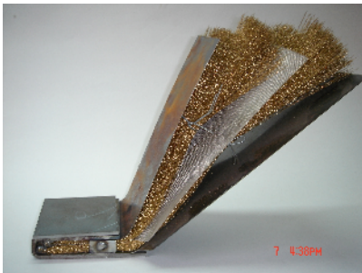
盾尾刷
