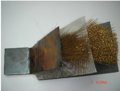
盾尾刷
