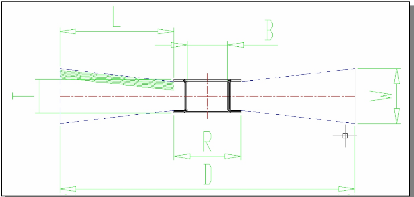
小直徑單片輪刷系列(所有尺寸皆可依客戶需求訂製)
